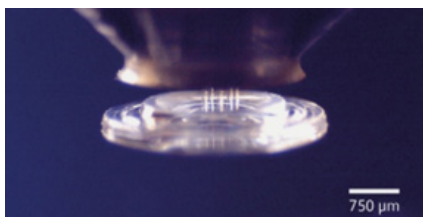
Adhäsiver Greifer zur Handhabung von Mikrolinsen
